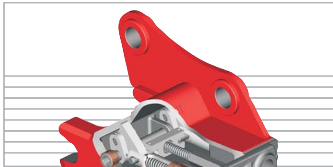
Verriegelungsmechanik geschützt im abgedichteten Gehäuse, Riegelbolzen eingefahren
