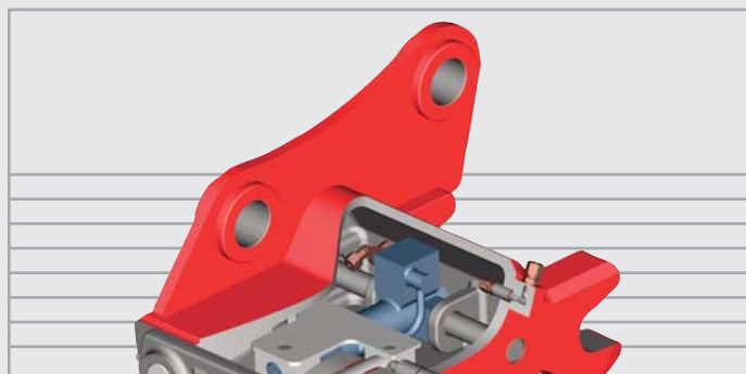
Hydraulikzylinder mit integriertem Sicherheitsventil, Schnellwechsler sicher verriegelt
